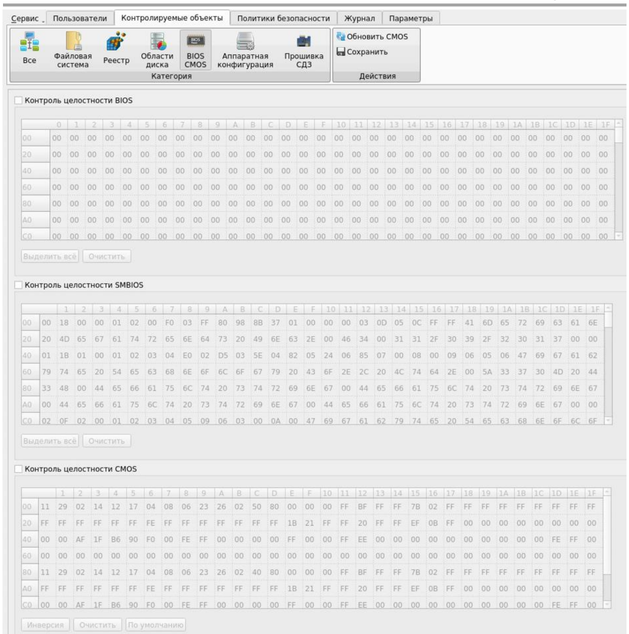
Рис. 2. Контроль BIOS/CMOS/SMBIOS
